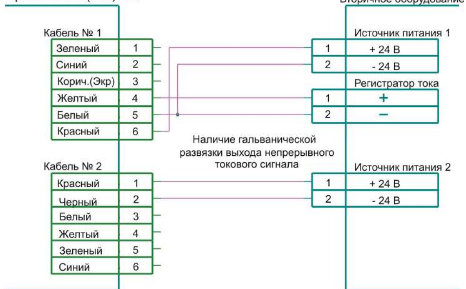
Рисунок Б.4 – Подключение цепей питания и выхода непрерывного токового сигнала
