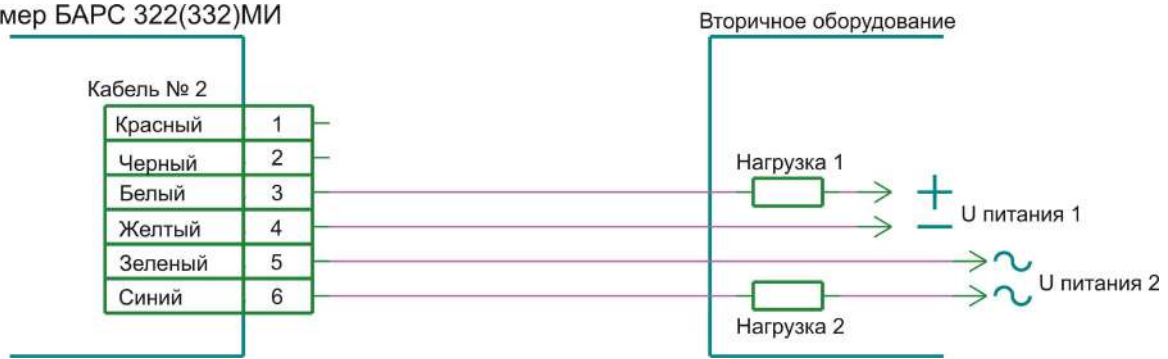
Рисунок Б.3 – Пример подключения цепей релейных выходов
