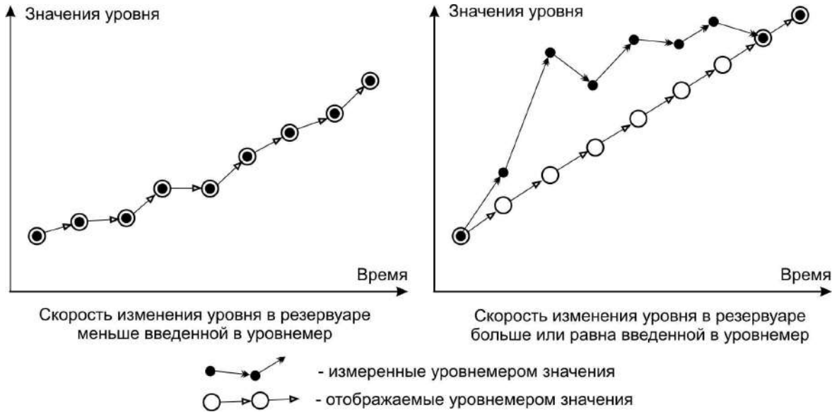
Рисунок 79 – Пример отображения результатов измерения
