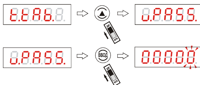
Рисунок 64 - Переход к вводу пароля пользователя
