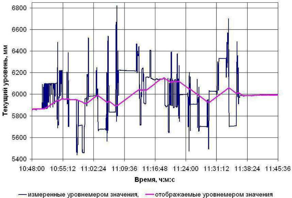
Рисунок 80 – Пример отображения результатов измерения
